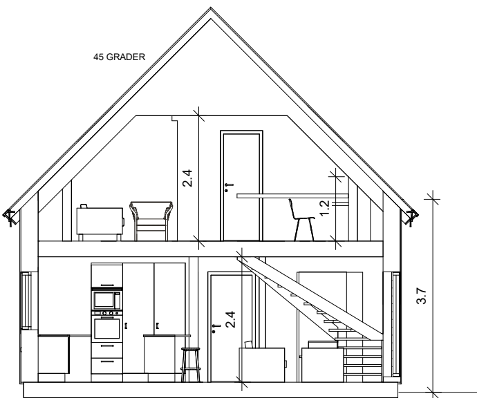
SEKTION A-A
